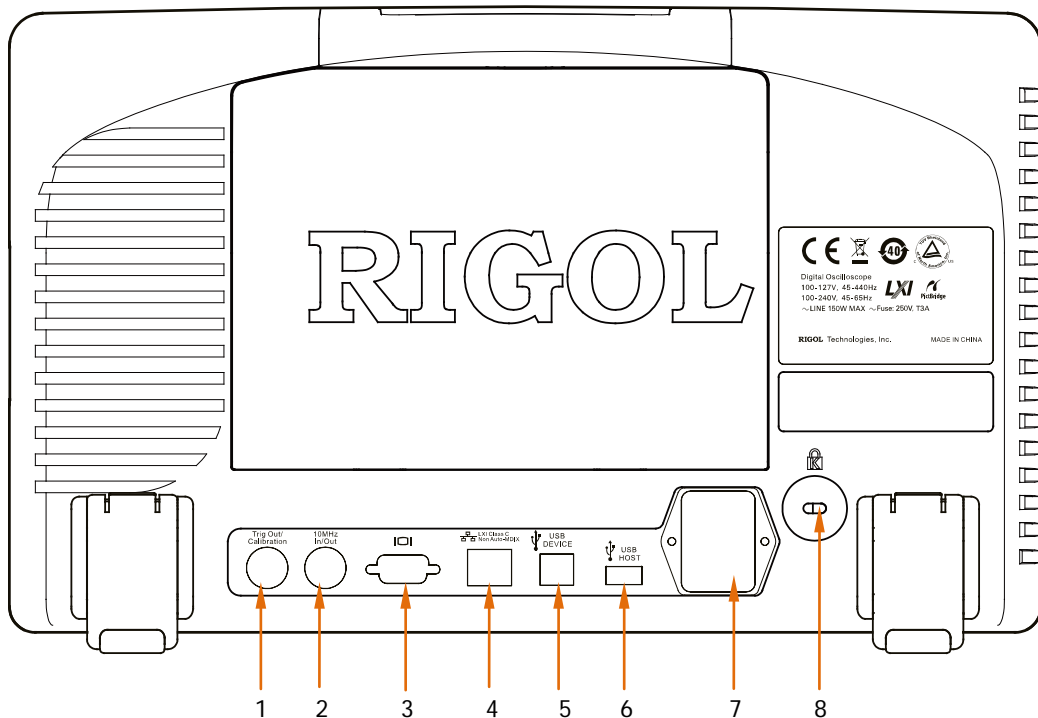
图 1-12 后面板总览
