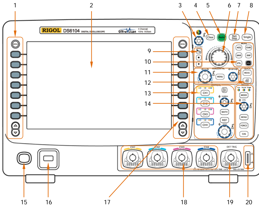
图 1-11 前面板总览
