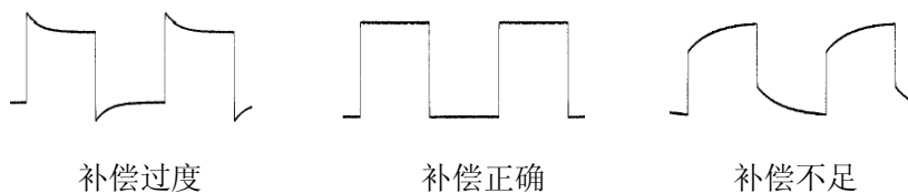
图 1-10 探头补偿
