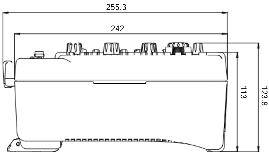
图 1-2 侧视图
