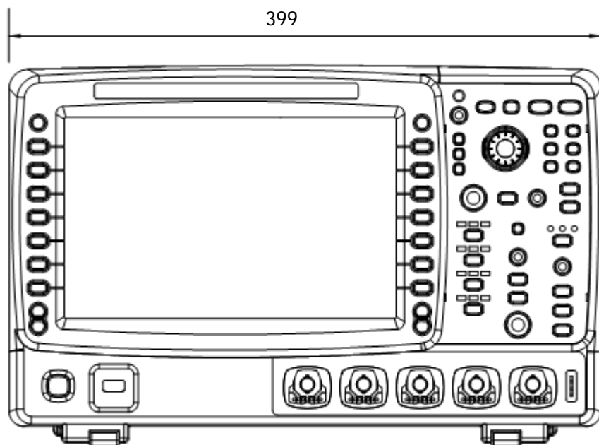
图 1-1 正视图
