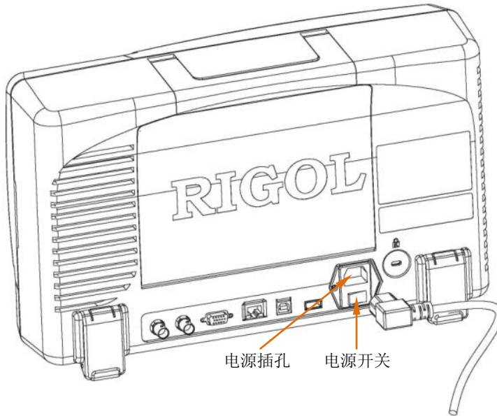
图 1-5 连接电源
