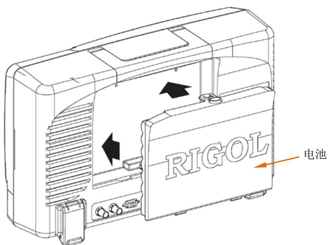
图 1-6 安装电池
