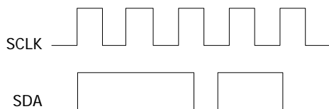
图 8-10 SPI 串行总线
