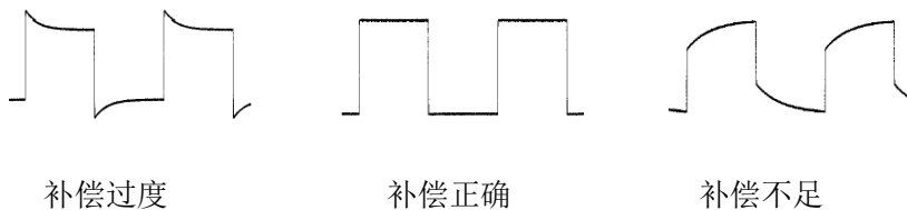
图 1-9 探头补偿
