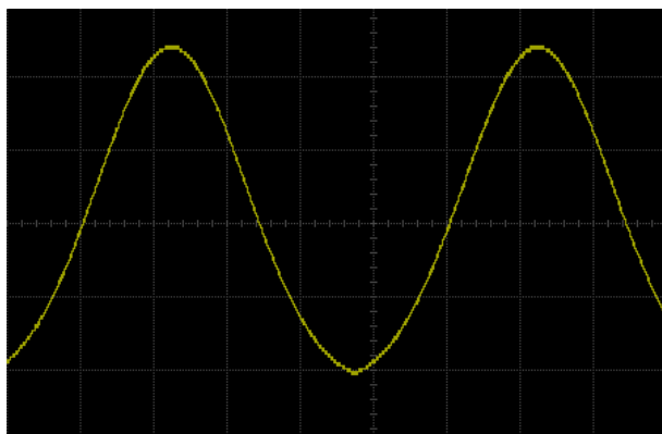
图 13-6 高斯函数波形示意图
