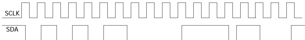
图 8-5 I2C 串行总线
