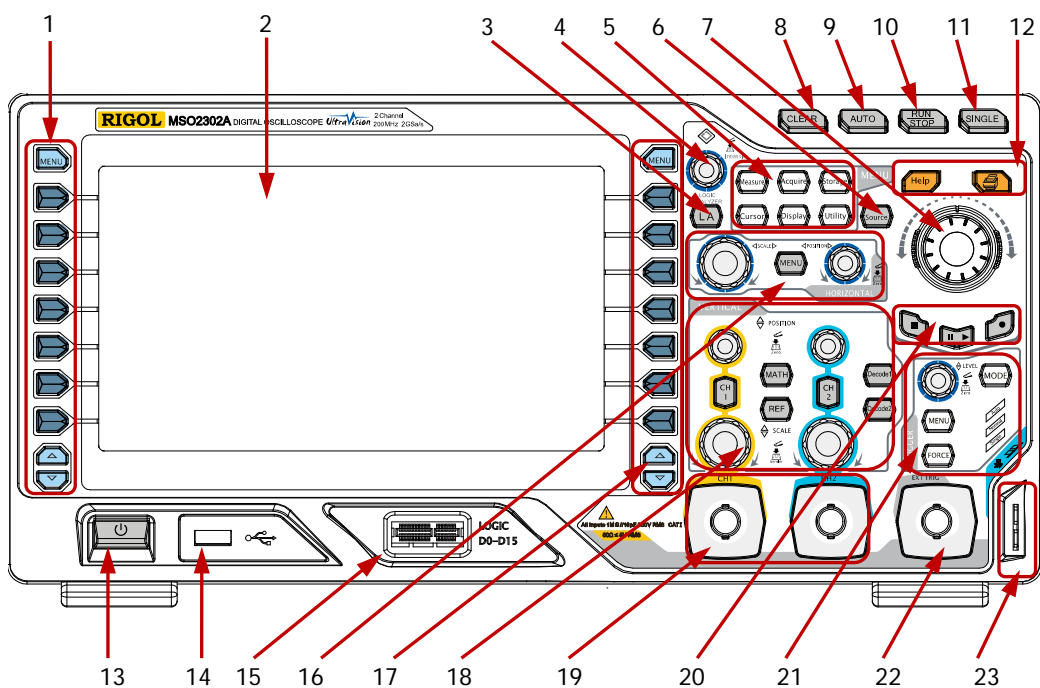
图 1-10 前面板总览
