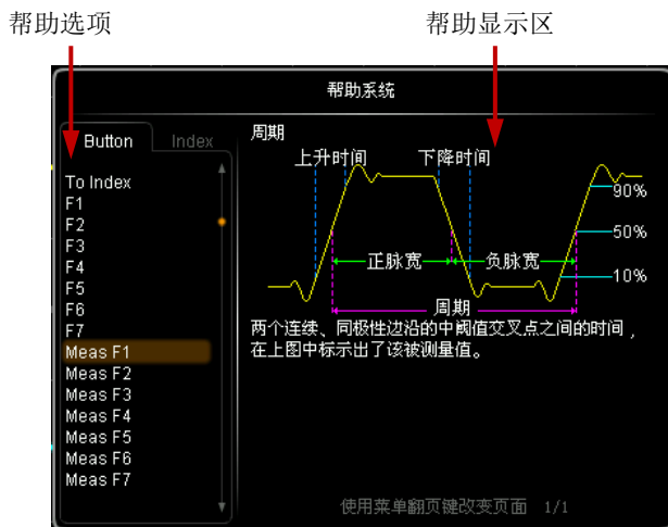
图 1-14 帮助界面
