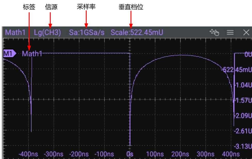
图 9.5 运算结果显示窗口
