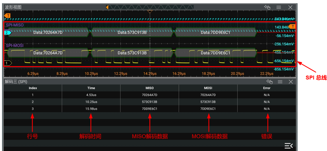
图 21.12 SPI 解码事件表
