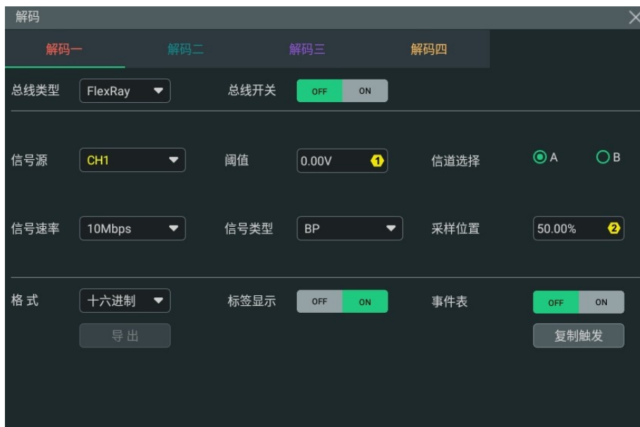
图 21.20 FlexRay 解码菜单
