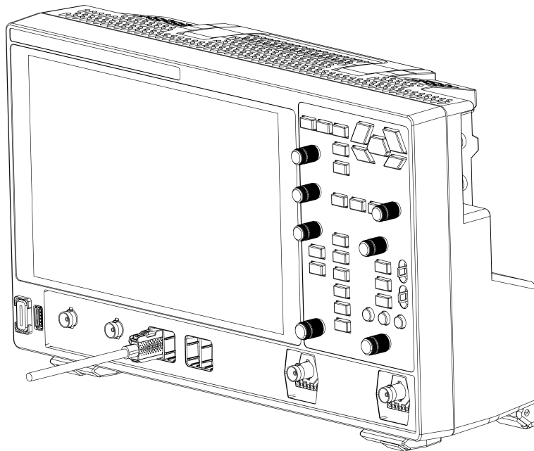
图 4.11 连接逻辑探头
