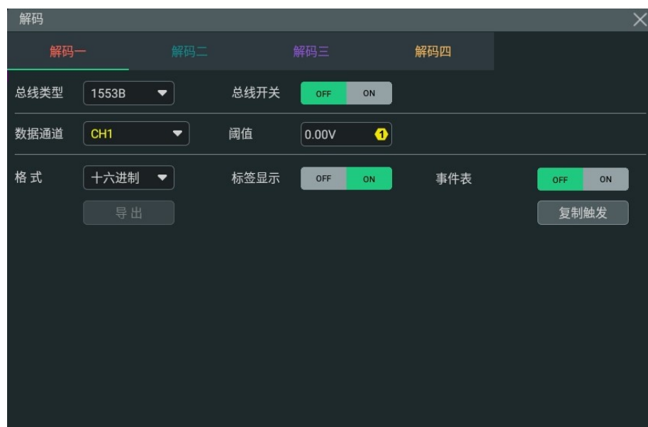
图 21.23 1553B 解码菜单
