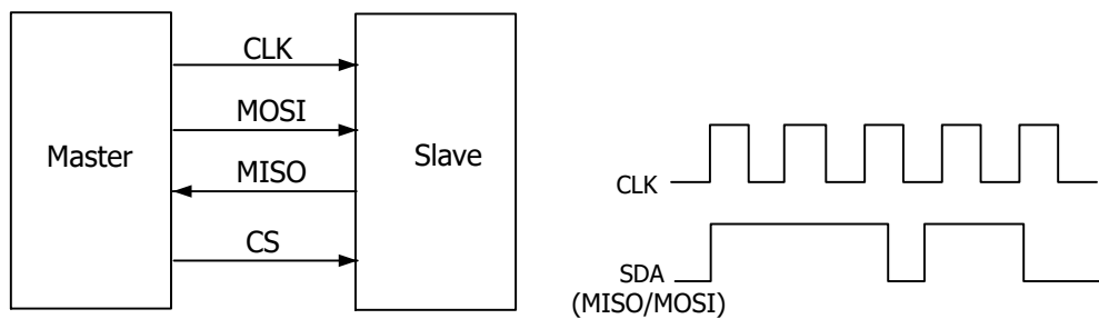
图 21.10 SPI 串行总线
