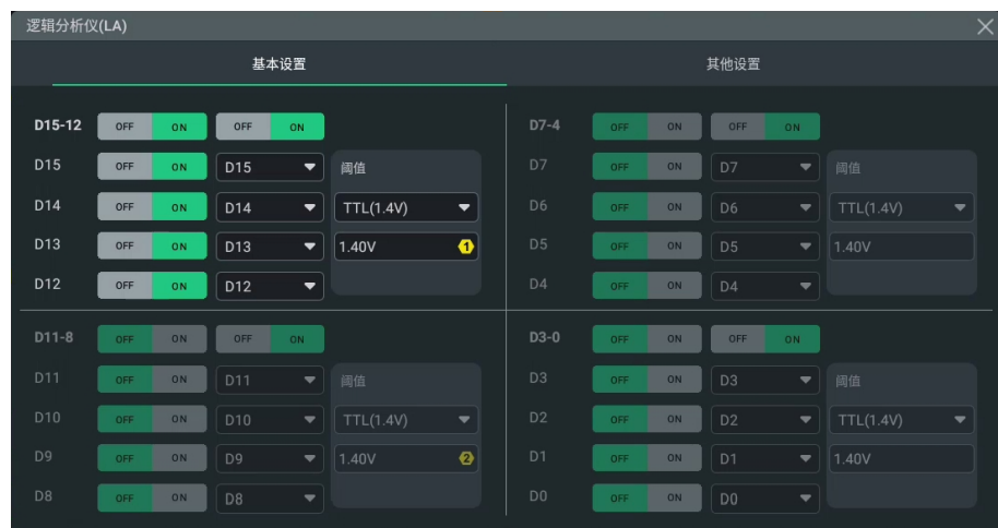
图 12.1 逻辑分析仪基本设置菜单
