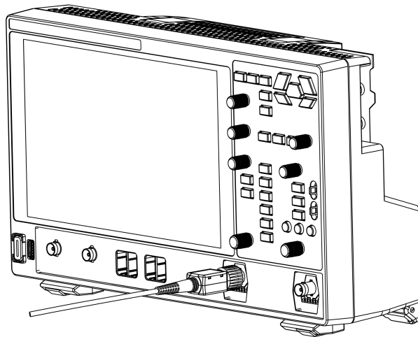
图 4.7 连接无源探头 (MSO 型号)
