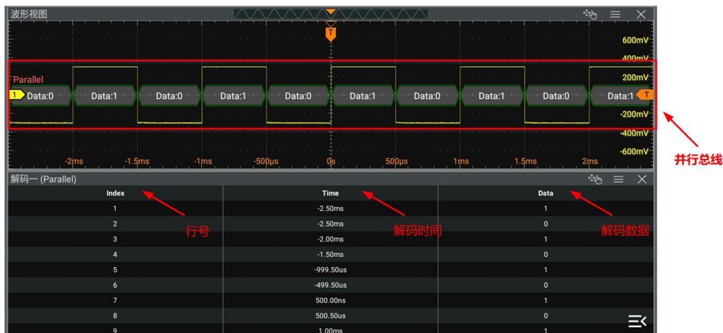
图 21.3 并行解码事件表
