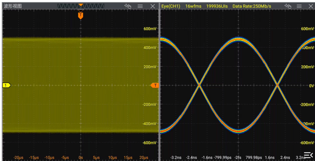
图 14.2 眼图测量窗口
