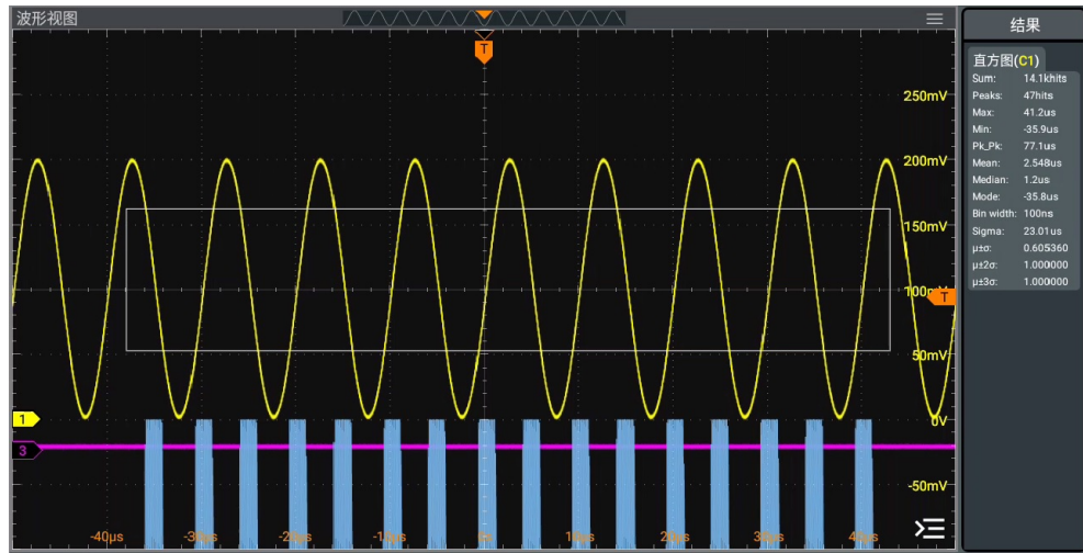
图 13.2 直方图分析界面
