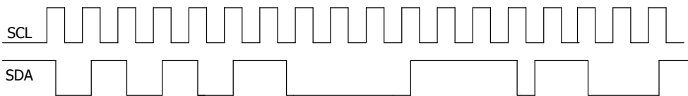
图 21.7 I2C 串行总线
