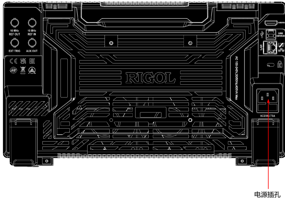
图 4.4 连接电源
