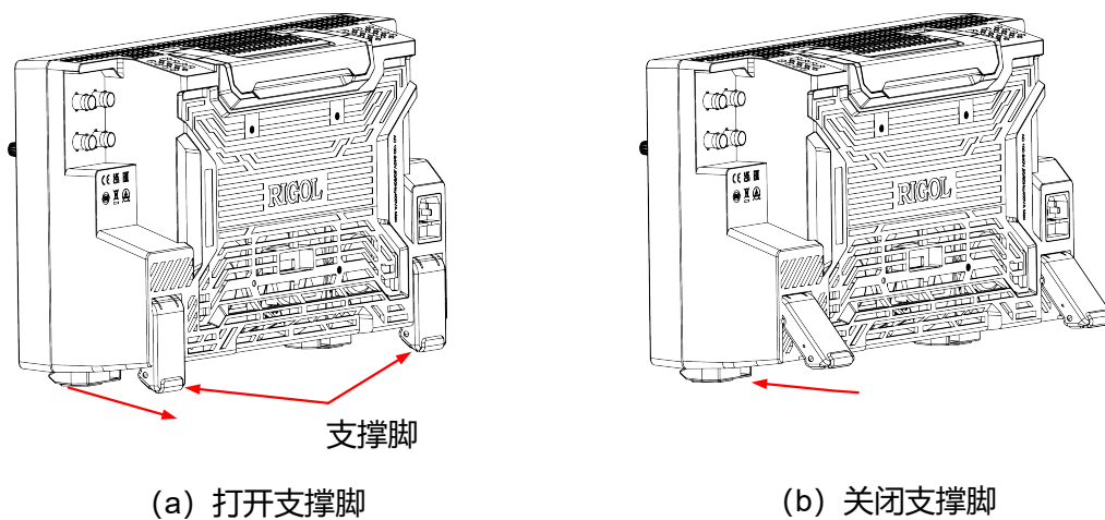
图 4.3 调节支撑脚
