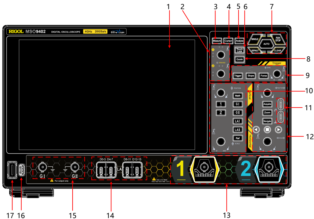
图 4.15 MSO9402 前面板
