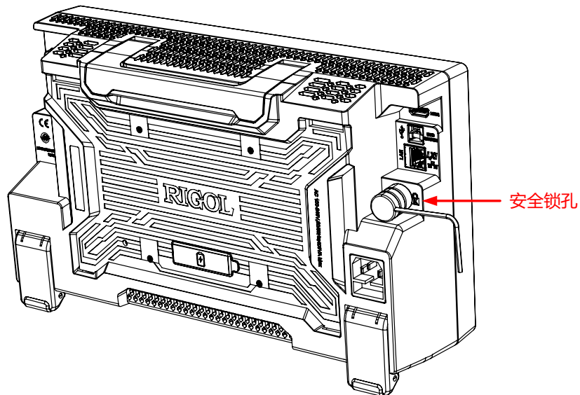
图 4.28 使用安全锁
