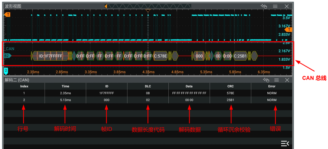
图 21.15 CAN 解码事件表
