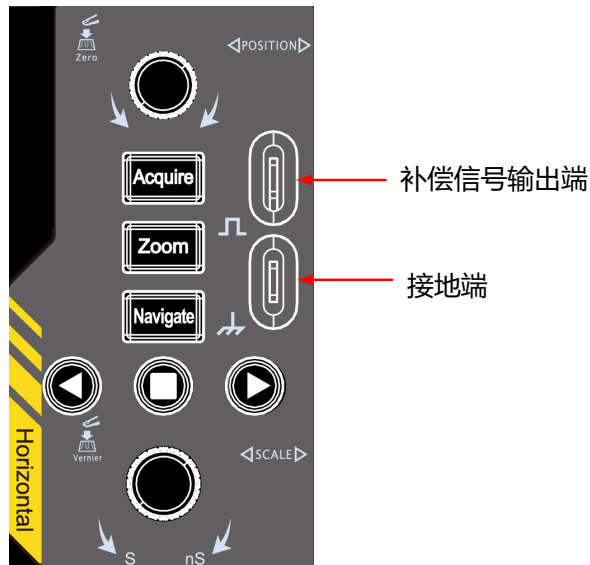
图 4.12 补偿信号
