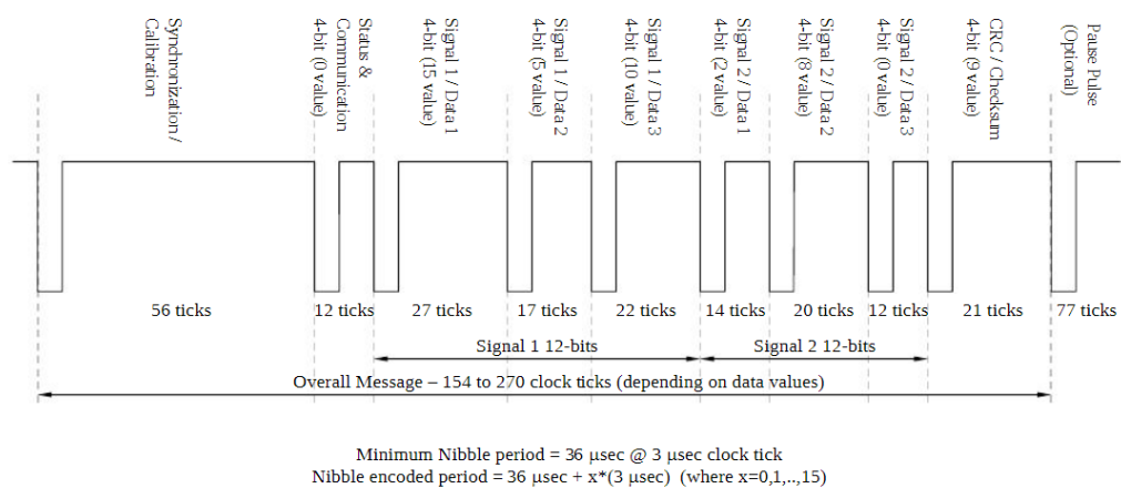
图 21.25 SENT 数据帧结构
