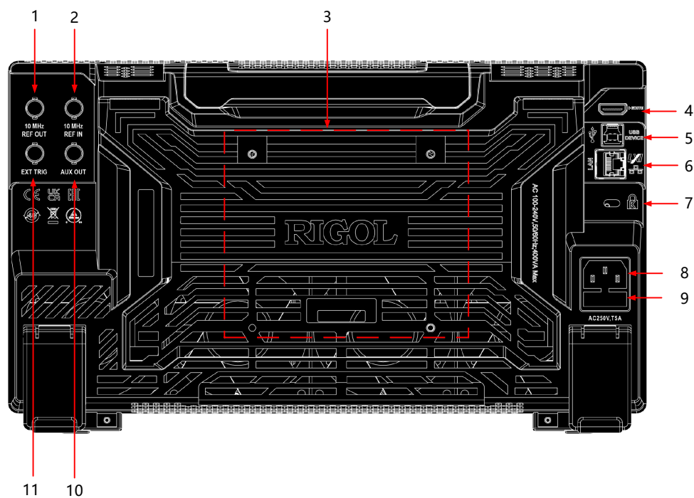
图 4.17 后面板
