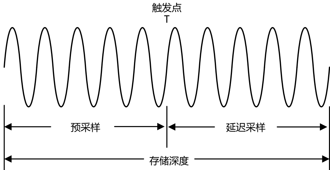
图 7.2 存储深度示意图
