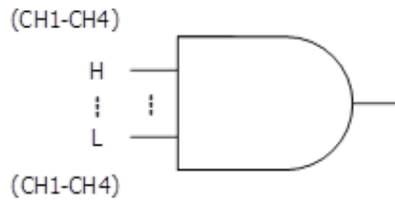
图 8.9 码型触发
