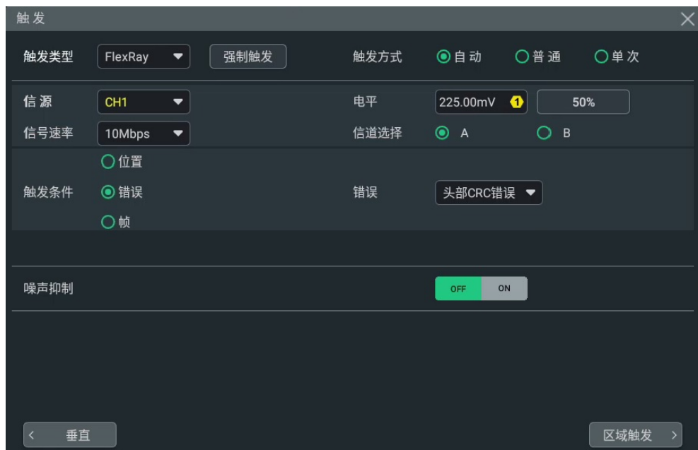
图 8.36 FlexRay 触发配置菜单
