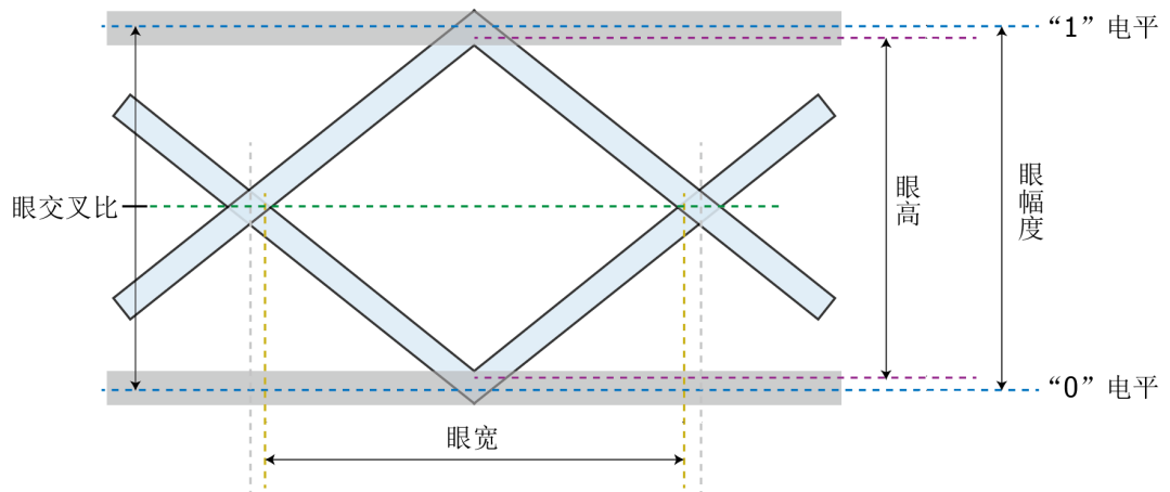
图 14.3 眼图参数示意
