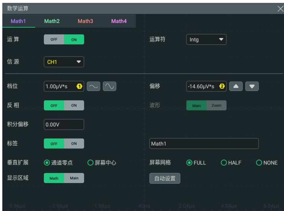
图 9.4 函数运算菜单
