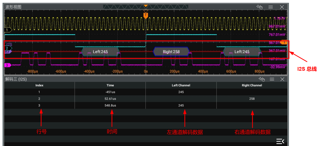
图 21.19 I2S 解码事件表
