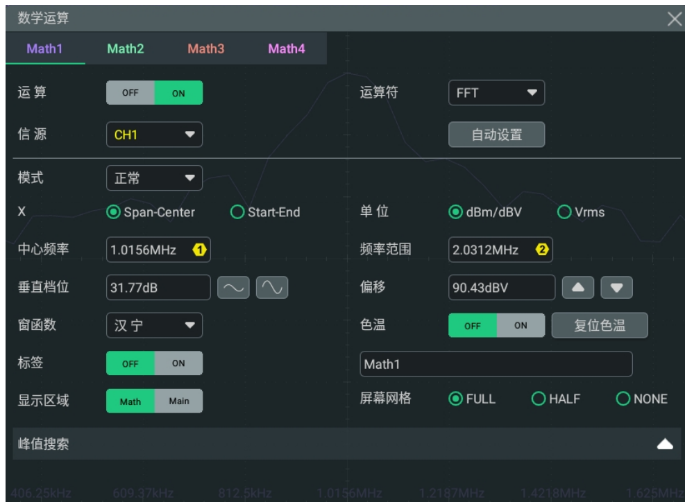
图 9.6 FFT 运算菜单
