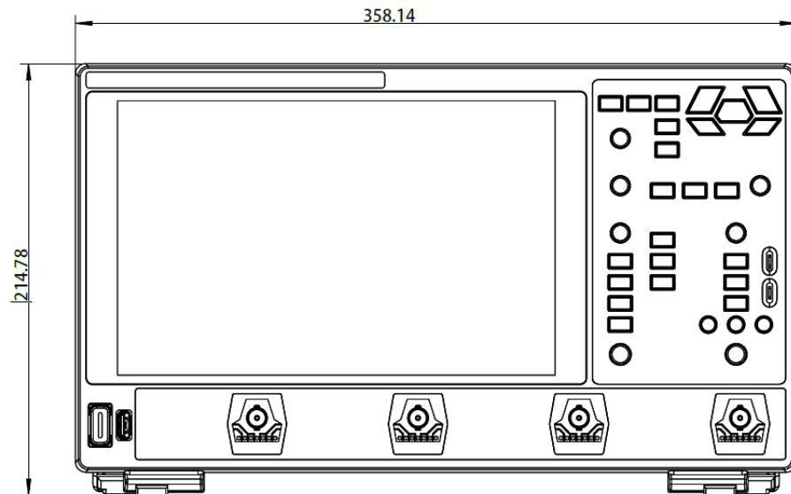
图 4.1 正视图
