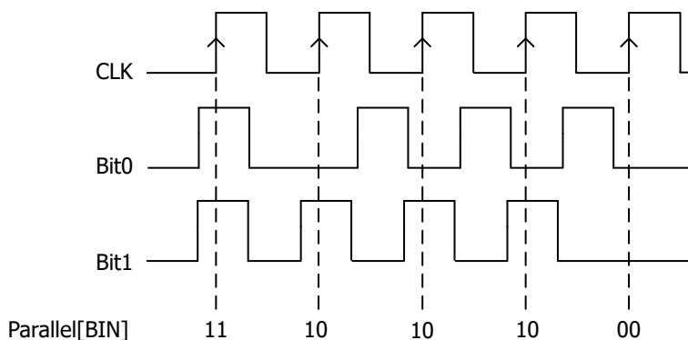
图 21.1 并行解码示意图
