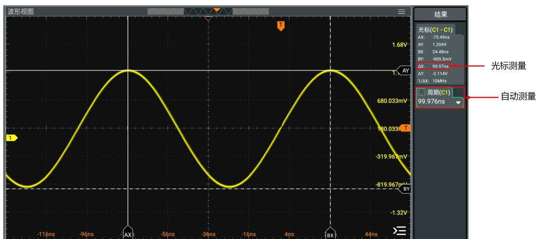
图 10.8 手动光标测量实例
