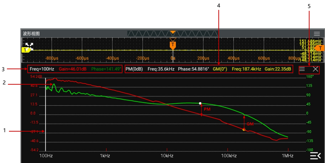
图 17.3 伯德图-波形显示
