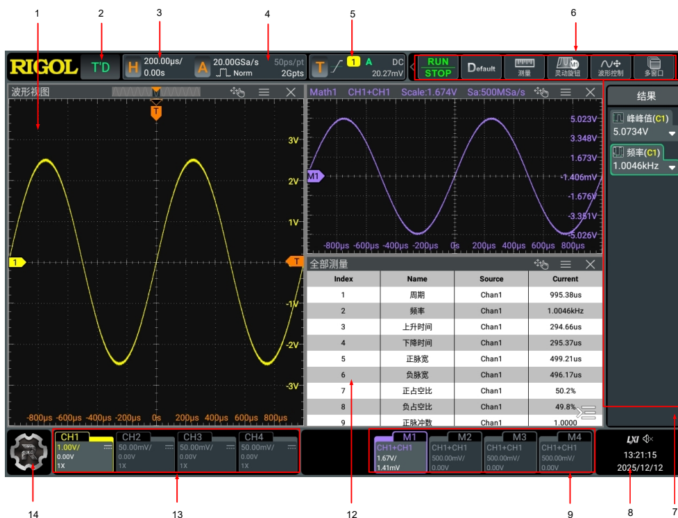
图 4.19 DS9404 用户界面
