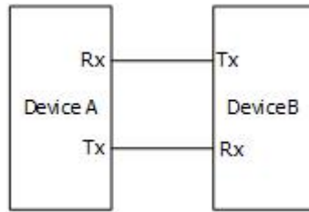
图 21.4 RS232 串行总线示意图
