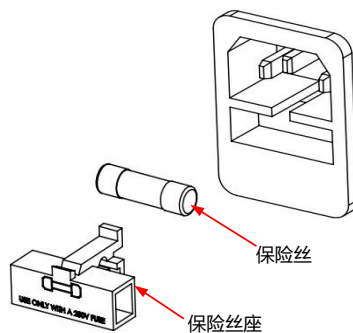
图 4.5 更换保险丝
