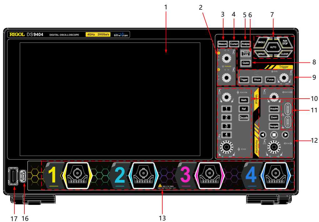
图 4.16 DS9404 前面板
