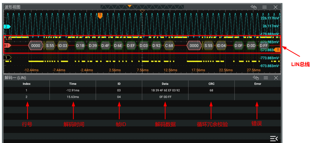
图 21.17 LIN 解码事件表
