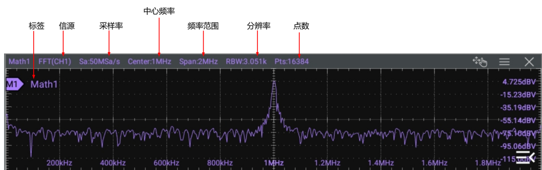
图 9.7 FFT 运算窗口
