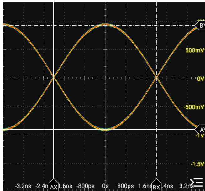
图 14.4 眼图光标
