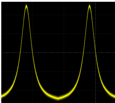
图 16.6 洛伦兹
