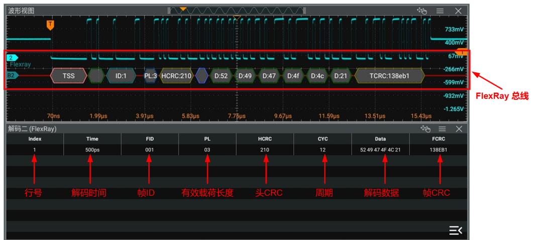
图 21.22 FlexRay 解码事件表
