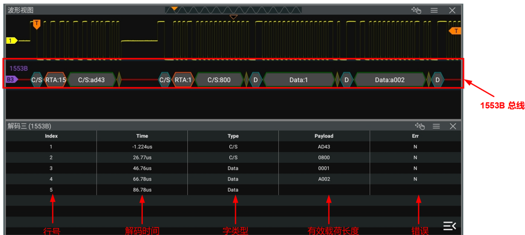
图 21.24 1553B 解码事件表
