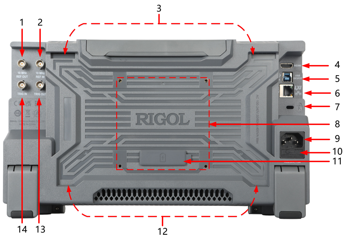
图 4.4 DNA5000 系列后面板
