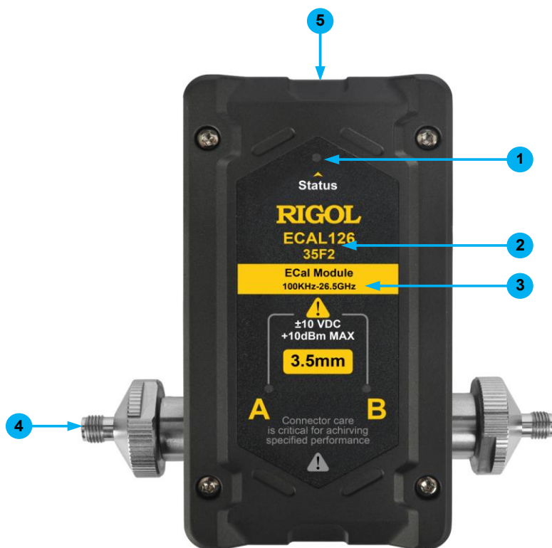
两端口 3.5 mm (阴头) 接口
