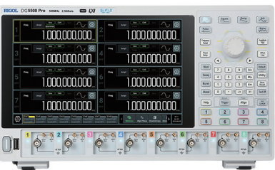
DG5000 Pro 系列函数 / 任意波形发生器
